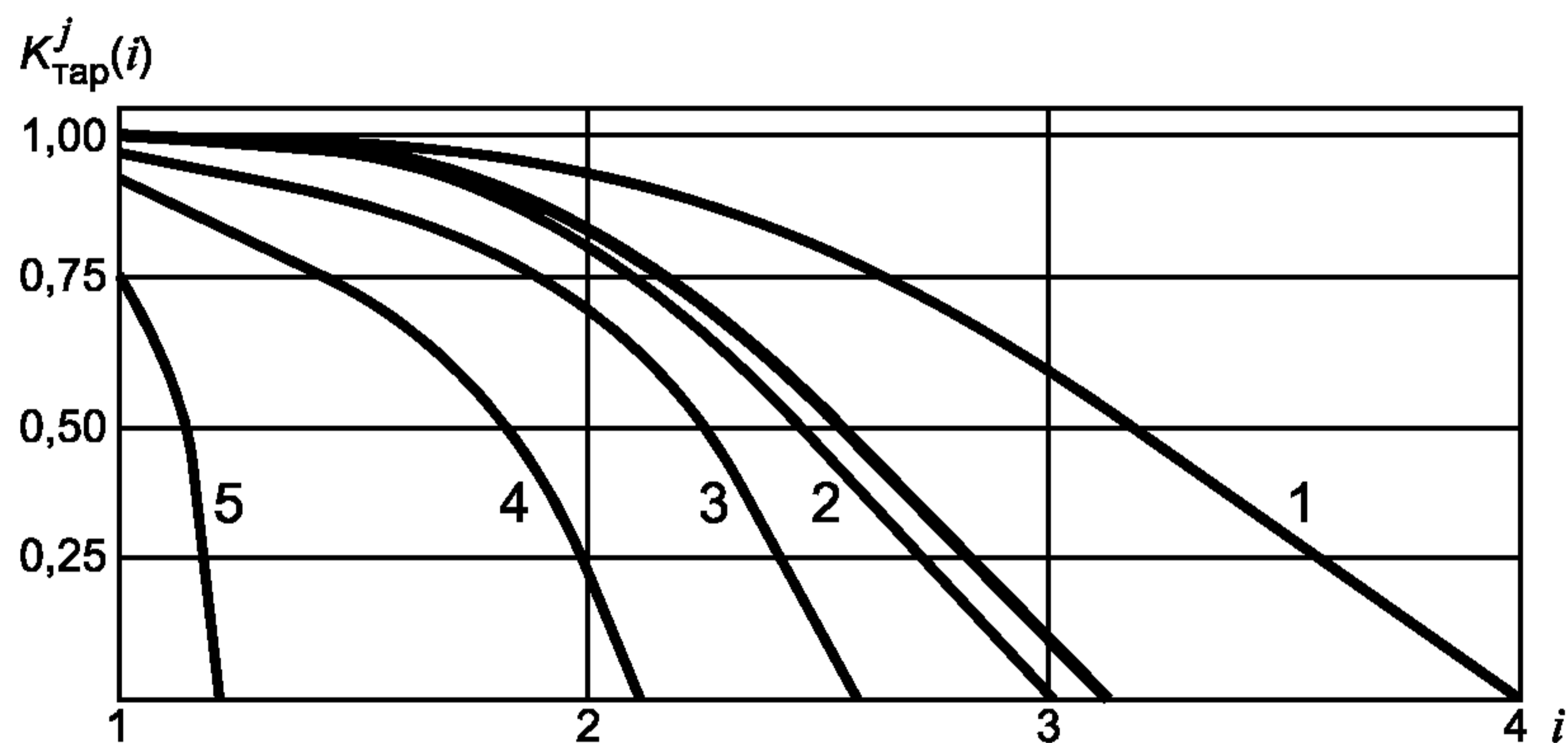
Рисунок 2 — Зависимость K^j(i) , нанесенная на серию тарифовочных кривых
