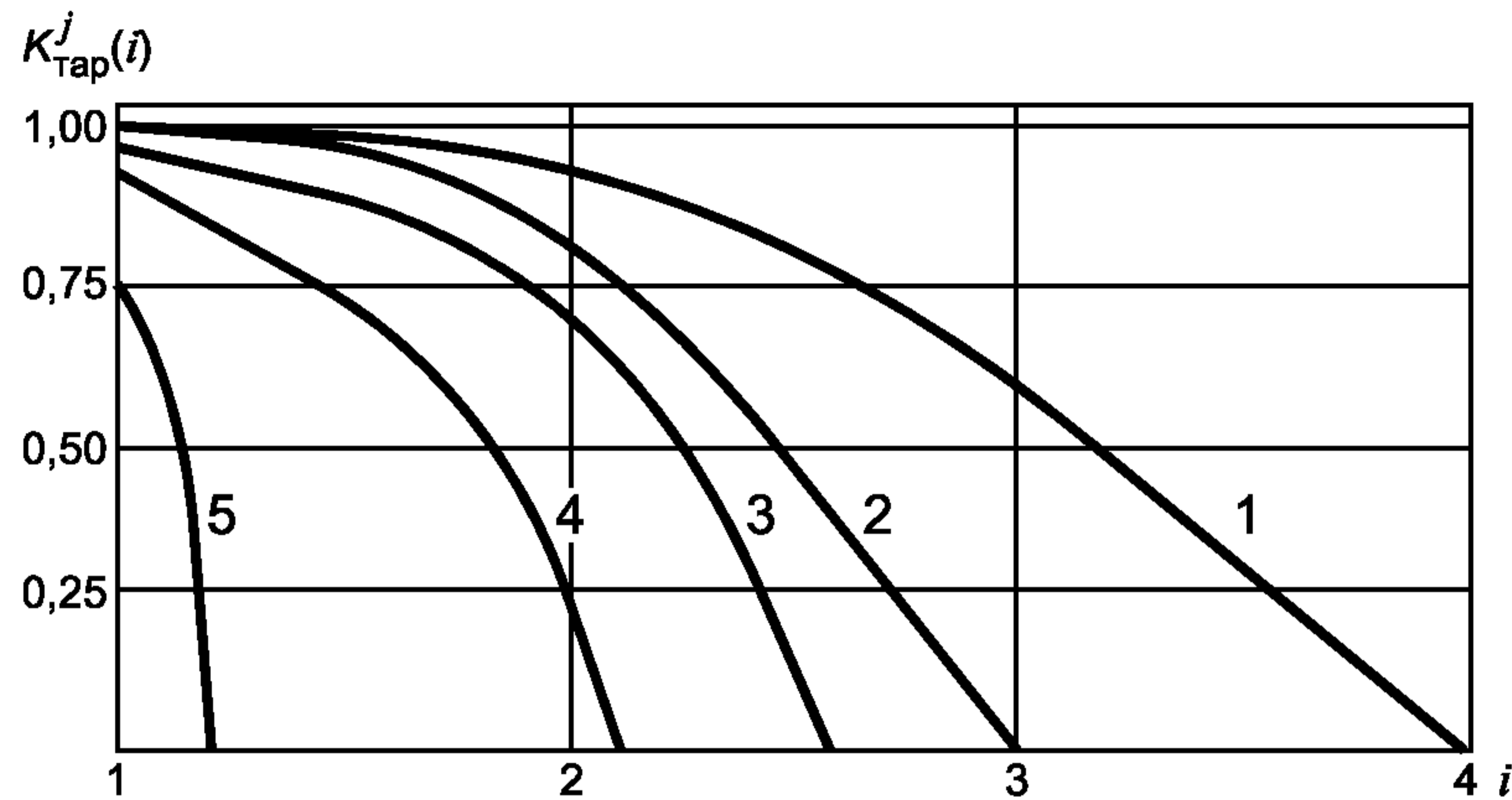
Рисунок 1 — Серия тарифовочных кривых K_{\text{тар}}^j(i)
